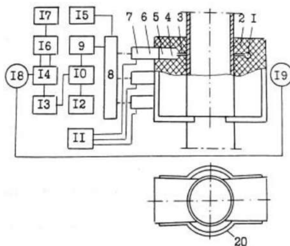
Рис.2. Блок-схема аппаратуры для определения насыщенности пористой среды жидкостью и газом методом гамма-скопии
