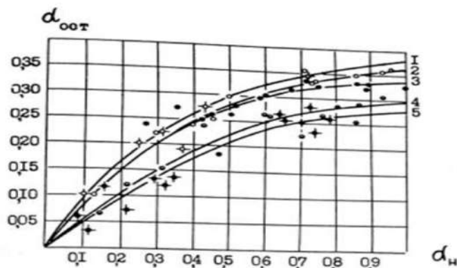
Рис. 1. Зависимости коэффициента остаточной газонасыщенности от коэффициента начальной газонасыщенности при вытеснении из образца пористой среда газа пресной водой (1, 4), конденсатом (2, 3) и пластовой водой (5) 1,3 - керн гидрофильный; 2,4 - керн гидрофобный
