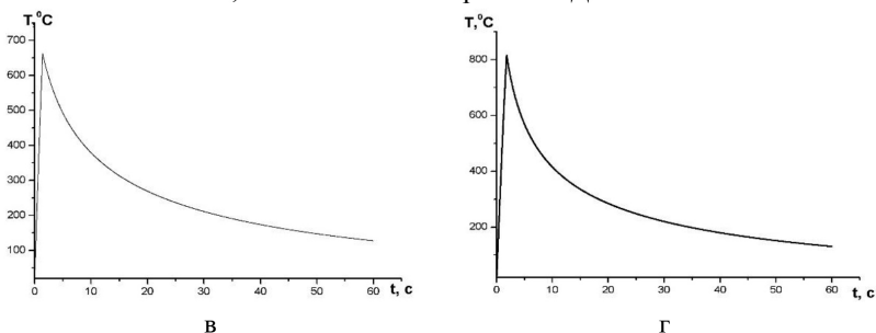
Рисунок 2. Зависимость температуры от времени при длительности импульса БТО 1,4 с и плотности энергии 200 Дж/см 2 (в), и 1,8 с при 255 Дж/см 2 (г).
