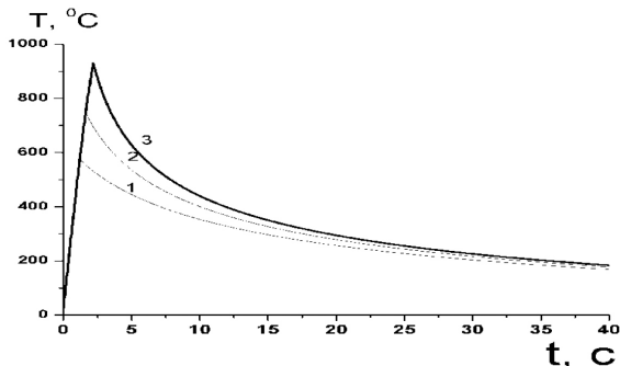
Рис. 1. Температурно-временные зависимости нагрева системы TiN/Ti/Si при импульсной фотонной обработке для различных плотностей энергии падающего излучения: (1) 170 Дж/см 2 , (2) 230 Дж/см 2 , (3) 285 Дж/см 2 .
