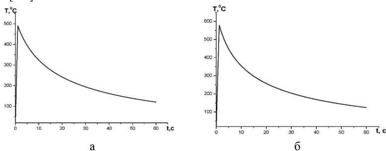
Рисунок 1.- Зависимость изменения температуры от времени при длительности импульса БТО 1,0 с и плотности энергии 142 Дж/см 2 (а), а также при длительности импульса БТО 1,2 с и плотности энергии 170 Дж/см 2
