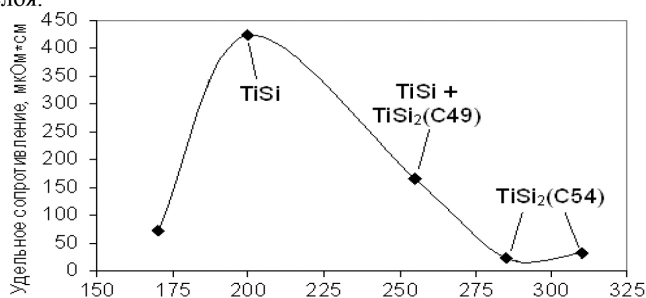
Рис. 2. Зависимость удельного электросопротивления силицидного слоя \text{Ti}_x\text{Si}_y и фазового состава от плотности энергии импульсной фотонной обработки.
